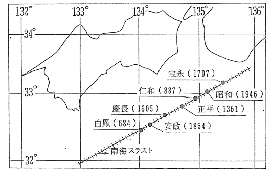
過去の南海地震の主震央位置と南海スラスト
